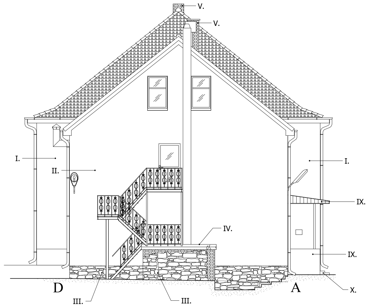
DA - ELEWACJA ZACHODNIA
