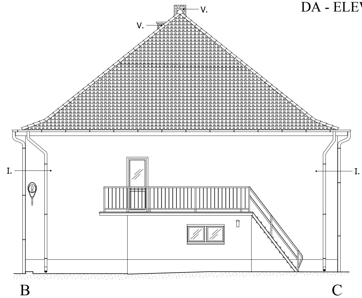
BC - ELEWACJA WSCHODNIA
